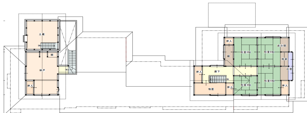
2階平面図
